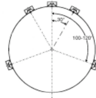
Figure 1. Disposition des haut-parleurs recommandés par la norme ITU-R BS.775.
